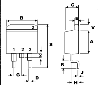
TO-263 (D2-PAK)
